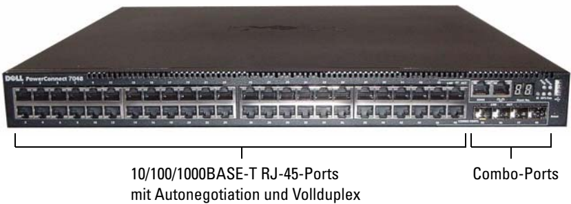
Abbildung 1-4. PowerConnect 7048 mit 48 10/100/1000BASE-T-Ports
